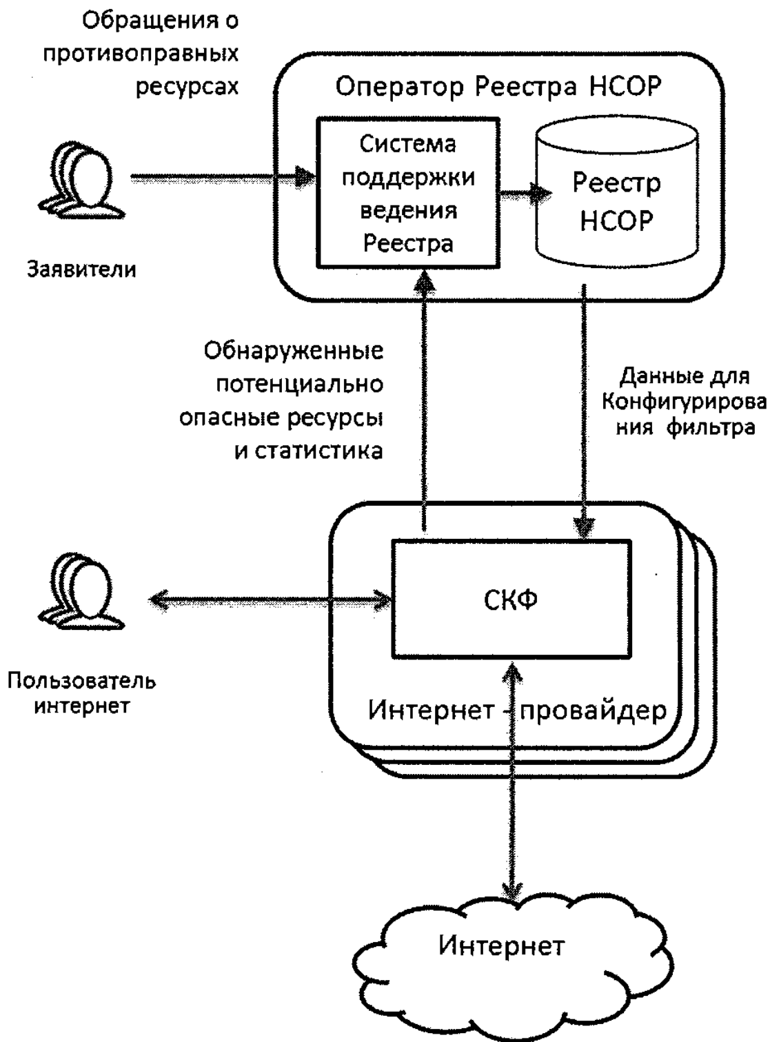
Рисунок 6. Принцип контроля доступа через Реестр NSCOP
